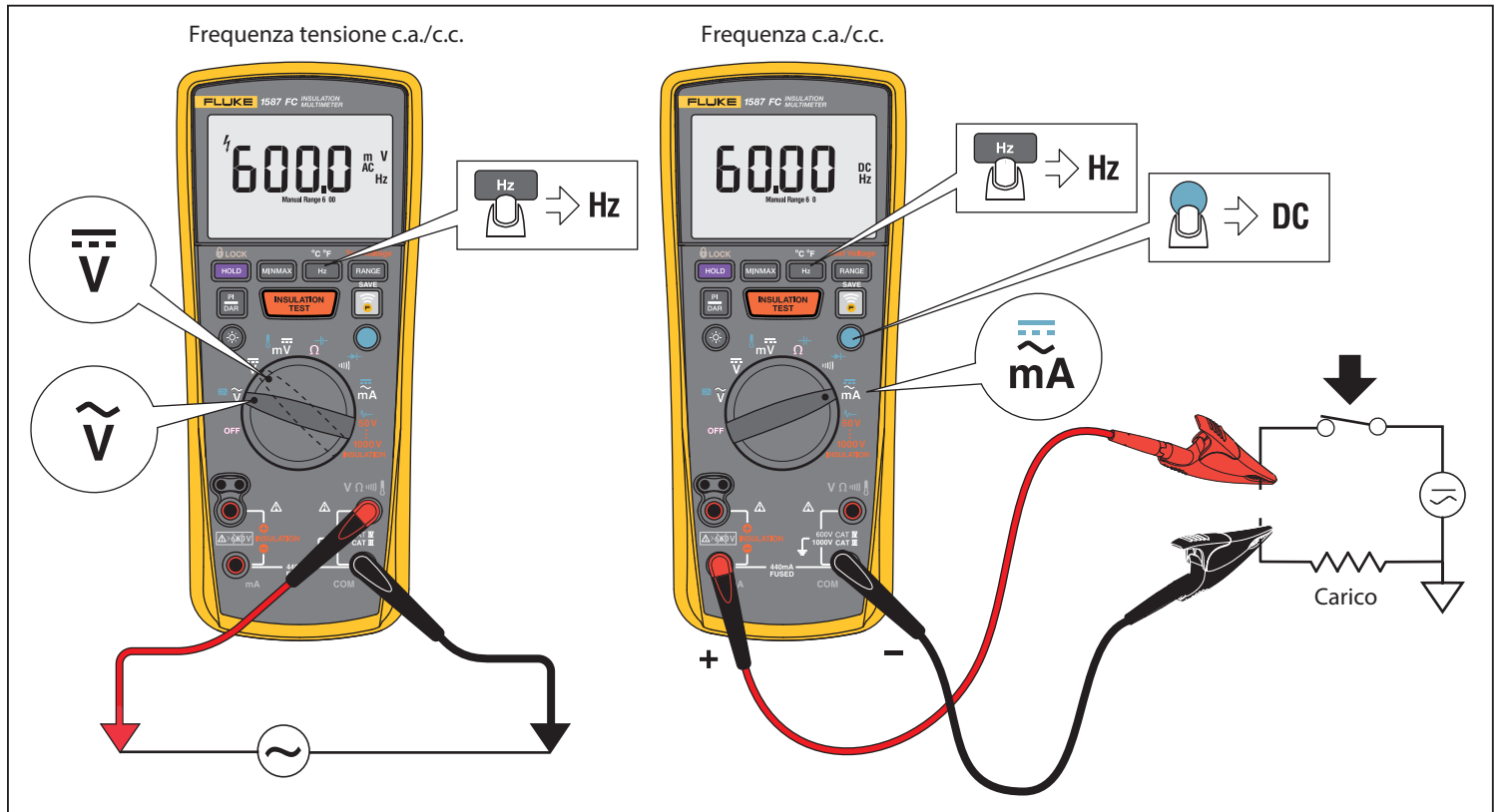
Figura 10. Misura della frequenza
