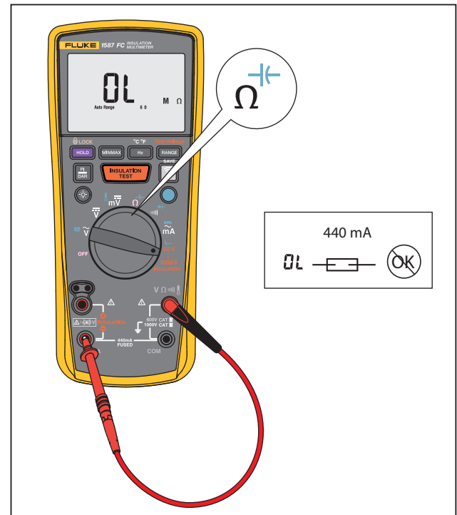
Figura 12. Verifica del fusibile
