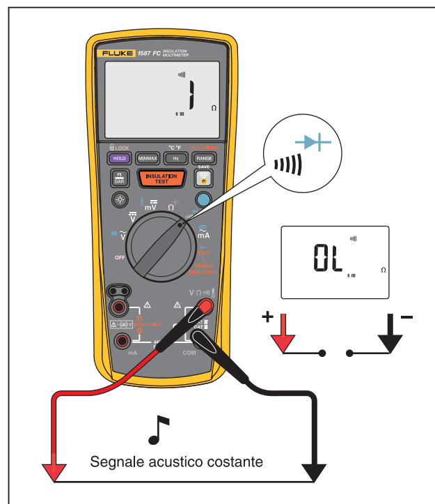
Figura 6. Test di continuità
