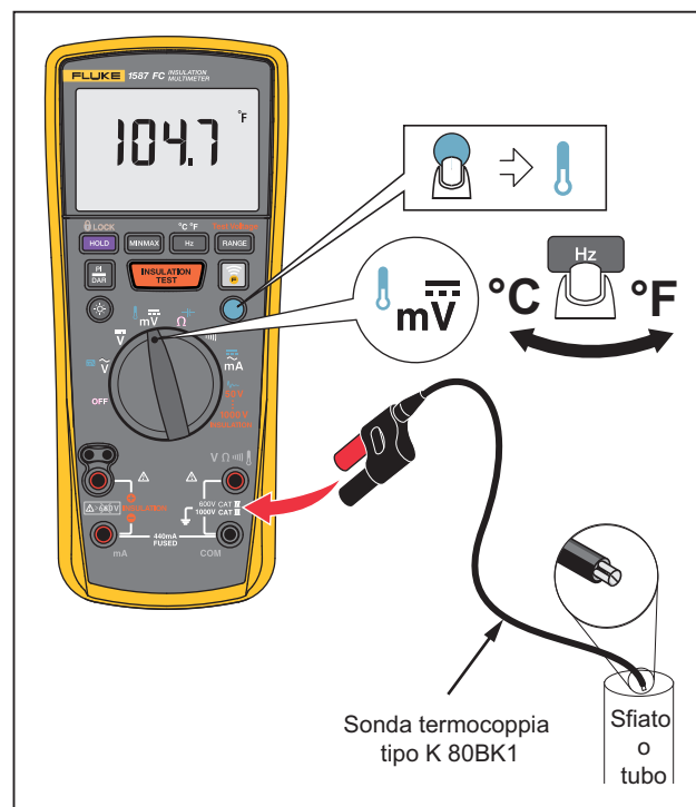
Figura 3. Misura della temperatura
