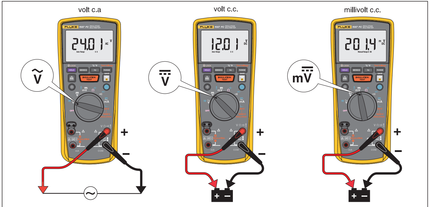
Figura 2. Misure di tensione c.a. e c.c.
