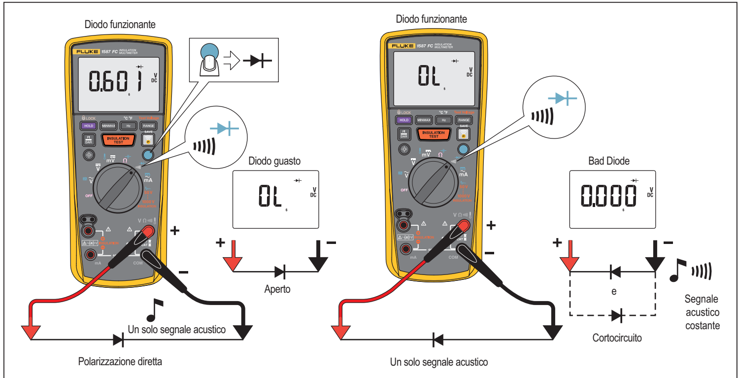
Figura 7. Test dei diodi
