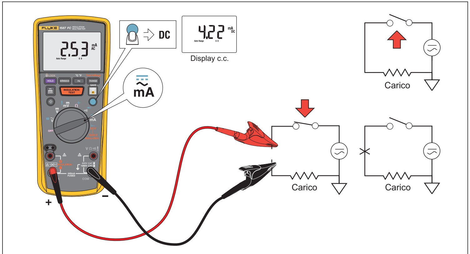
Figura 8. Misure di corrente c.a. o c.c.
