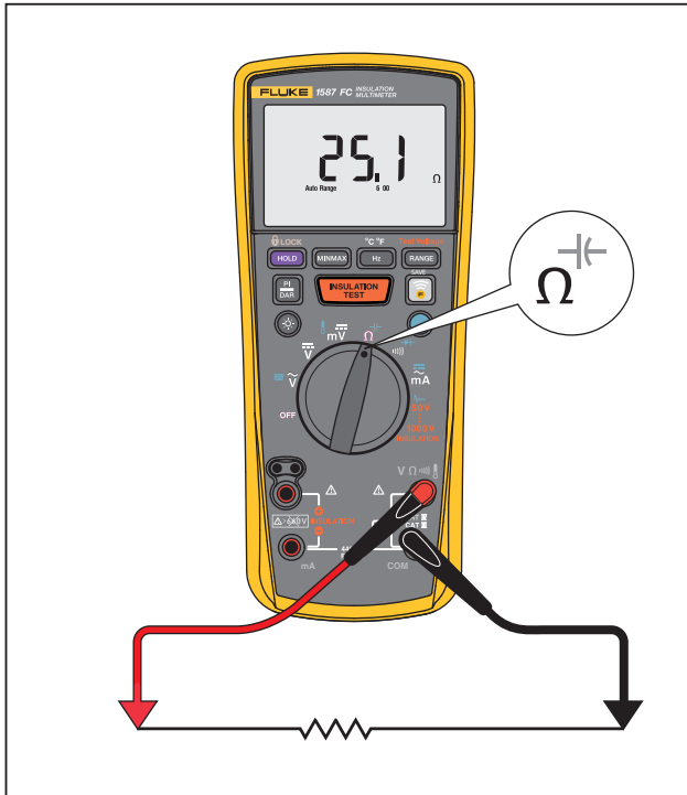
Figura 4. Misura di resistenza
