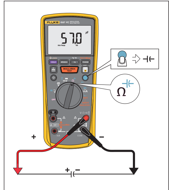
Figura 5. Misura di capacità
