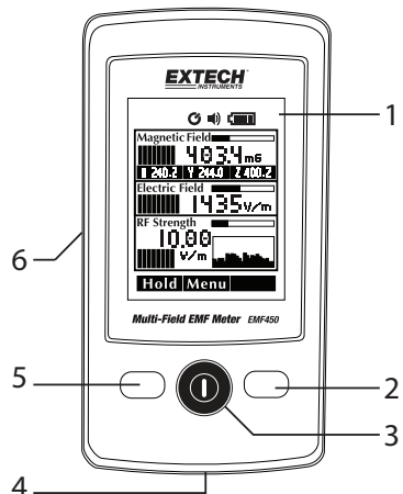
Figura 1 - Descrizione strumento
