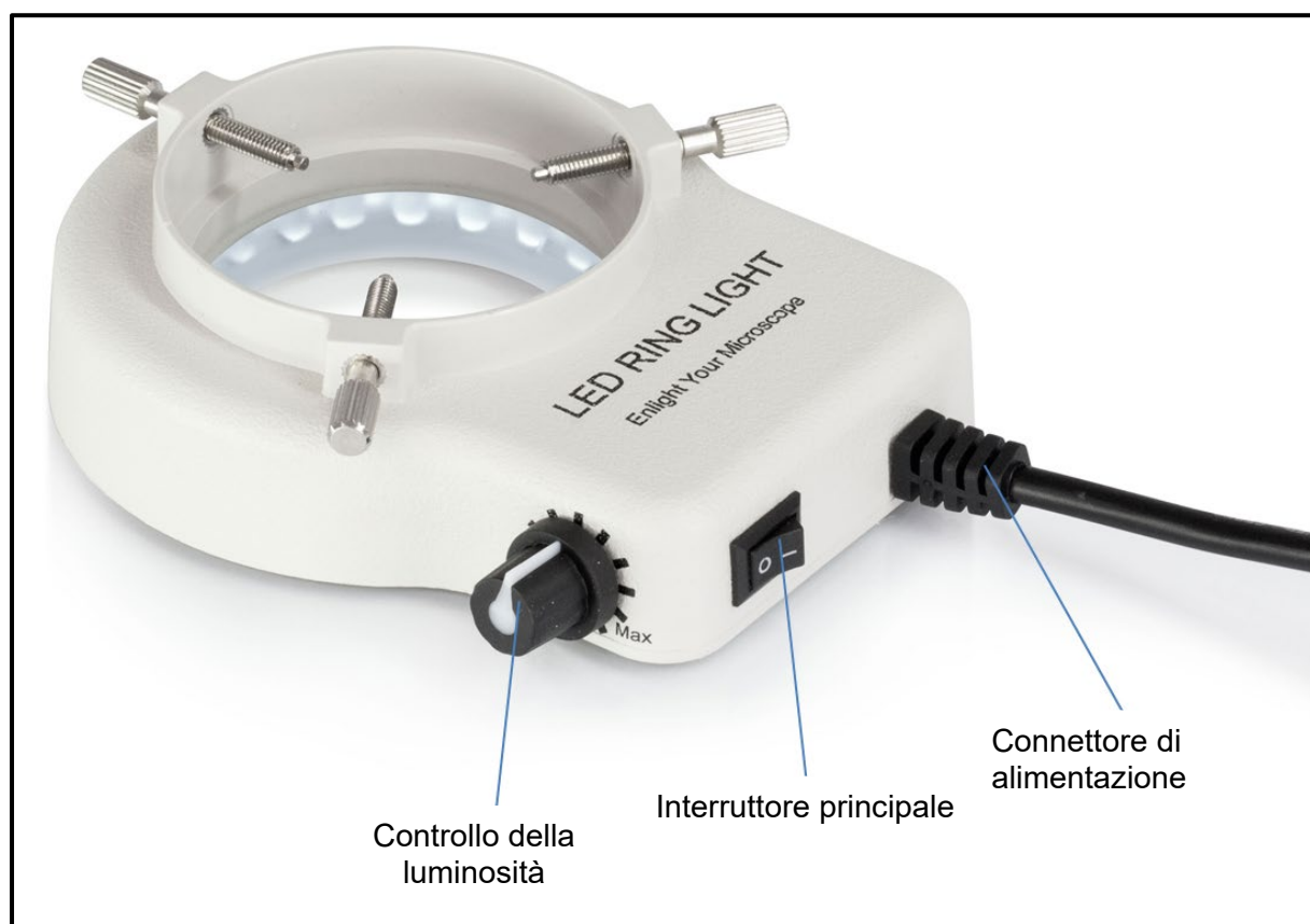
Controlli dell'illuminazione
