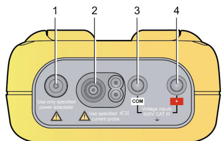
Figura 2: I morsetti nella parte superiore.
