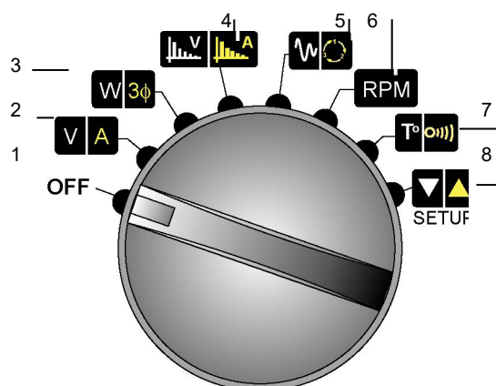
Figura 6: Visione delle modalità accessibili dal commutatore rotante.
