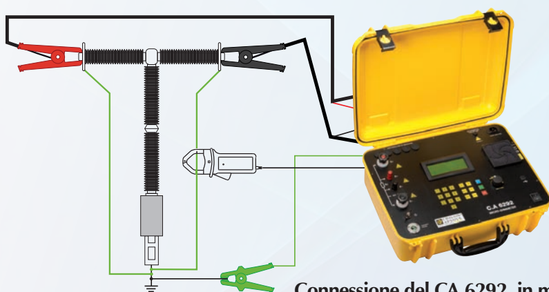
Connessione del CA 6292 in modalità BSG Utilizzo della pinza opzionale MR 6292.
