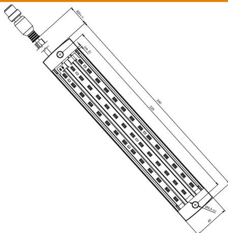
Disegno quotato
