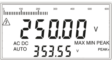
Esempio: misura di tensione su un azionamento elettrico
