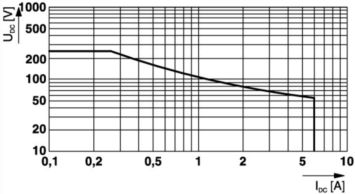
Relè curva di carico: carico ohmico
