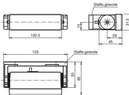
Misure di montaggio della staffa girevole
