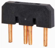
Ponte di stella, per DILM17-32
