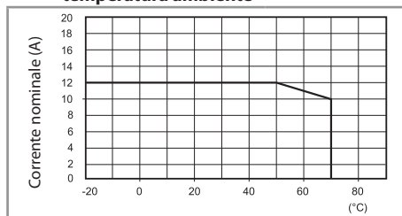
L 96 - Corrente nominale in funzione della temperatura ambiente
