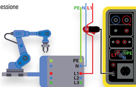
Schermata misurazione correntemp di dispersione differenziale tramite pinza opzionale G72
