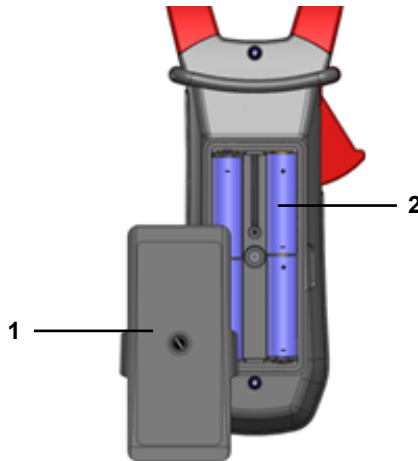
Figura 6: lo sportello d'accesso alle pile
