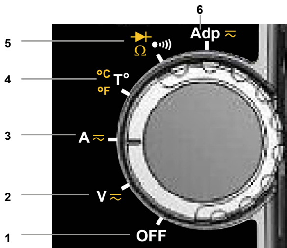
Figura 2: il commutatore
