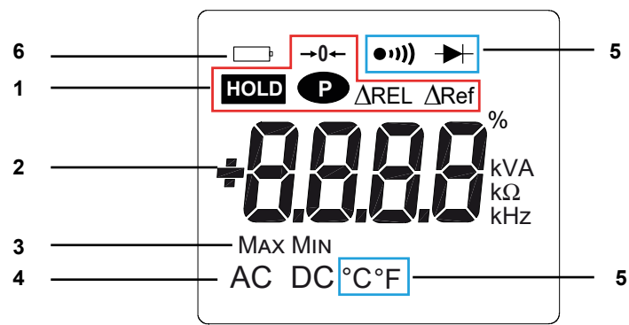
Figura 4: il display
