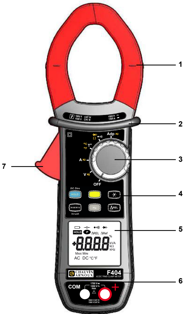
Figura 1: il multimetro a pinza F404
