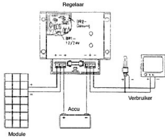
Afb. 2 Aansluitpunten
