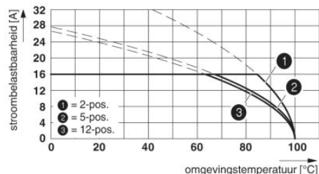
Deratingcurve voor: MSTB 2,5 HC/...-ST met MSTBVA 2,5 HC/...-G
