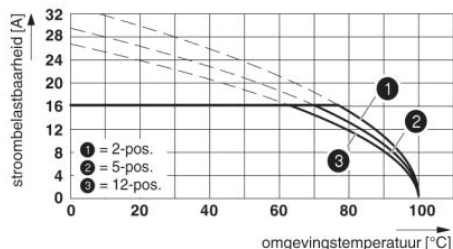
Deratingcurve voor: MSTB 2,5 HC/...-ST met MSTBA 2,5 HC/...-G
