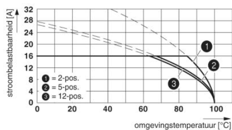
Deratingcurve voor: MSTB 2,5 HC/...-ST met MSTBVA 2,5 HC/...-G
