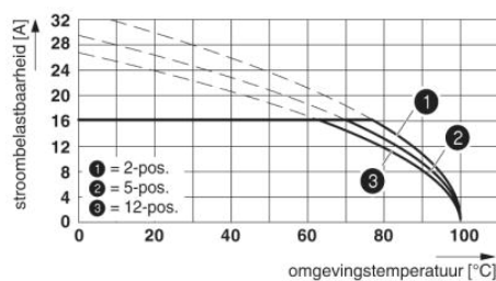
Deratingcurve voor: MSTB 2,5 HC/...-ST met MSTBA 2,5 HC/...-G
