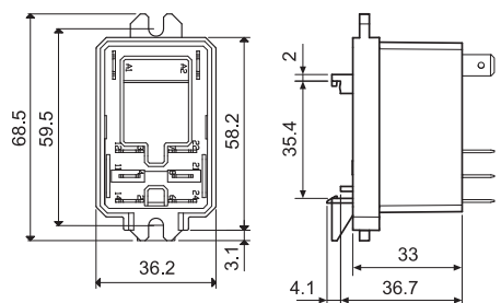
066.07 met relais
