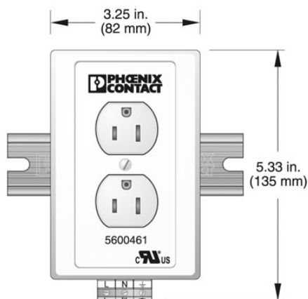
Vooraanzicht
