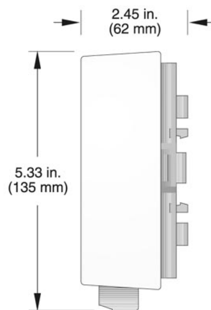
Zijaanzicht
