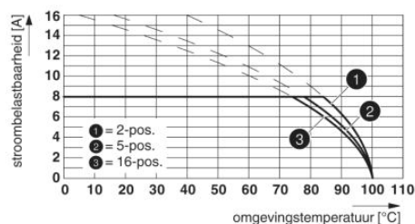
Type: MC 1,5/...-STF-3,81 met DFK-MC 1,5/...-GF-3,81 (met soldeeraansluiting)
