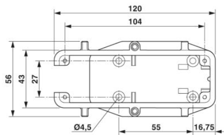
Maatschets bovenaanzicht
