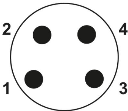
Poolschema steker M8, 4-polig, aanzicht stiftzijde
