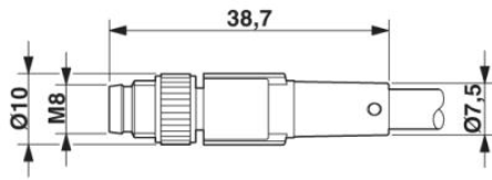
Steker M8 x 1, recht, afgeschermd
