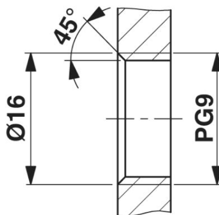
Behuizingsuitsparing voor Pg9-bevestigingsschroefdraad, Montagewand met schroefdraad
