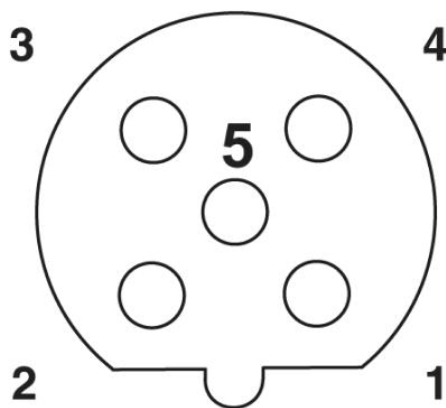
Poolschema bus M12, 5-polig, B-gepolariseerd, buszijde
