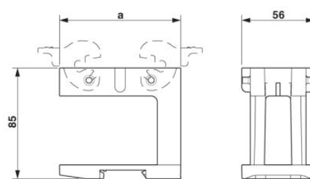
Maatschets, a = 93,5 mm
