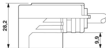
Steker M12 x 1, haaks
