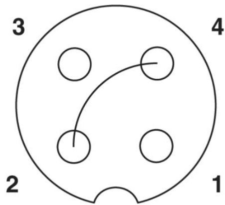
Poolschema bus M12, 3-polig, pin 2+4 doorverbonden, A-gepolariseerd, aanzicht buszijde
