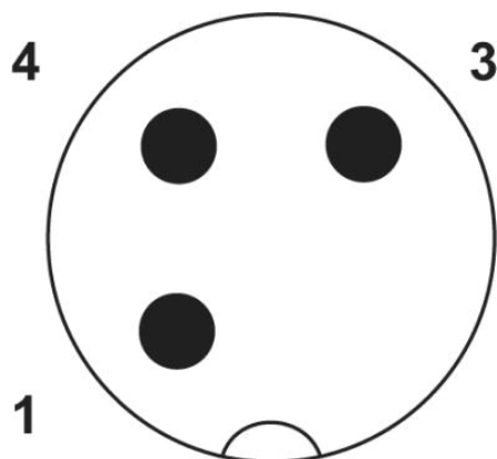
Poolschema steker M12, 3-polig, A- gepolariseerd, aanzicht stiftzijde
