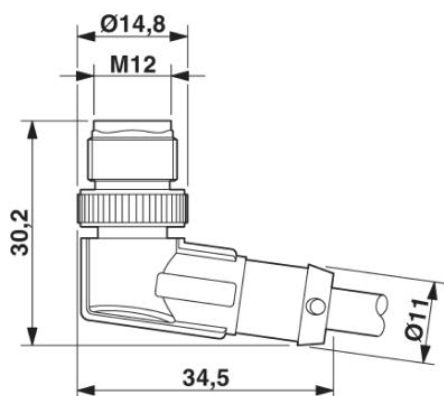
Steker M12 x 1, haaks
