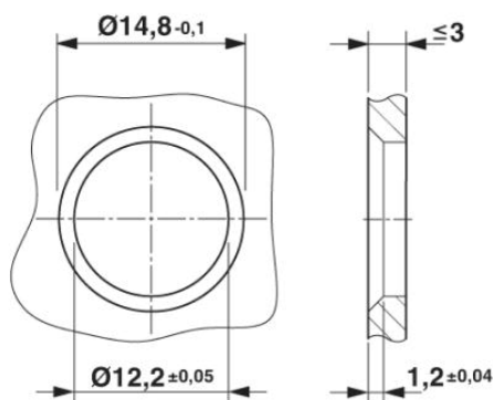
Behuizingsuitsparing voor 2-delige M12-inbouwconnector, met THR- en golfsoldeeraansluiting, variant 1
