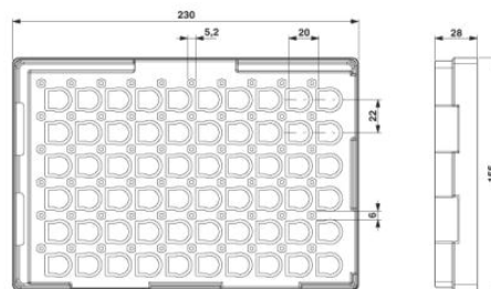
THR-tray-verpakking
