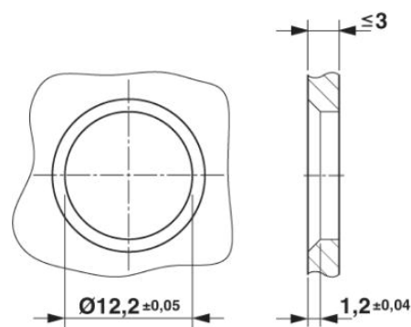
Behuizingsuitsparing voor 2-delige M12-inbouwconnector, met THR- en golfsoldeeraansluiting, variant 2
