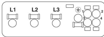
Poolschema aansluitzijde
