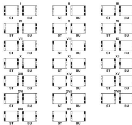
Polarisatieschema
