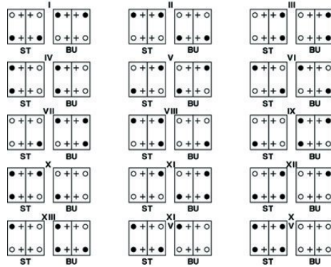
Polarisatie voor behuizingen met twee contactblokken
