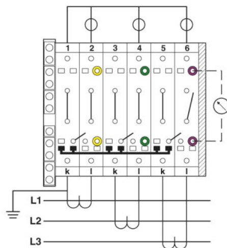
Driefase meettransformator-testschakeling
