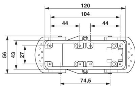
Maatschets bovenaanzicht
