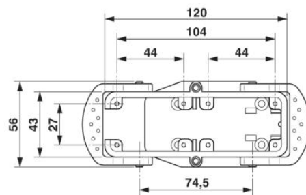
Maatschets, a = 120 mm
