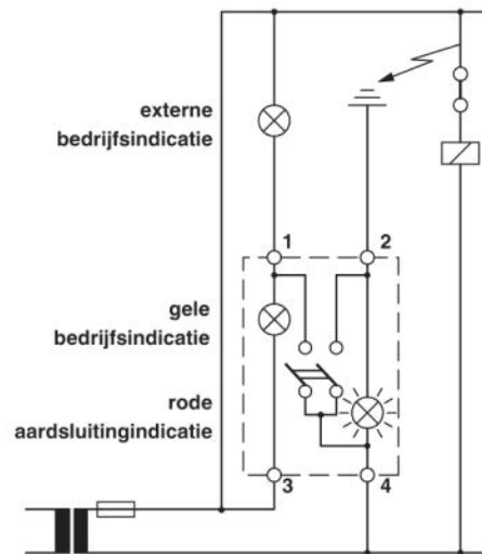
Aardsluiting
