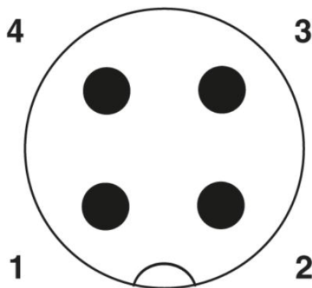
Poolschema stiftconnector M12 Y, 4-polig, A-gepolariseerd, aanzicht stiftzijde
