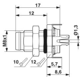
M8-inbouwstiftconnector
