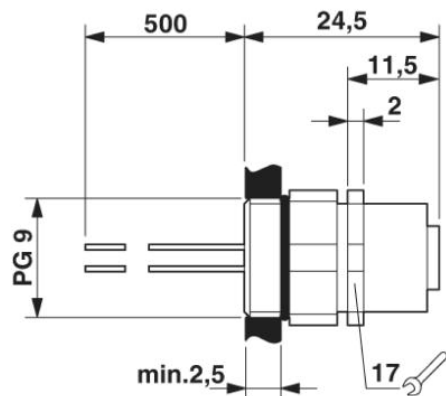
M12-inbouwbusconnector, positioneerbaar
