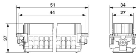
Buscontactblok
