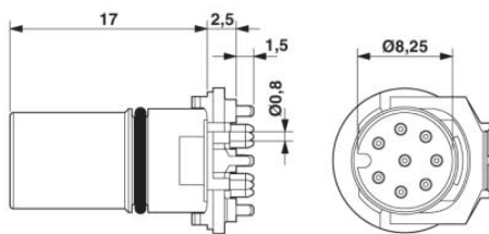
M12-buscontactblok
