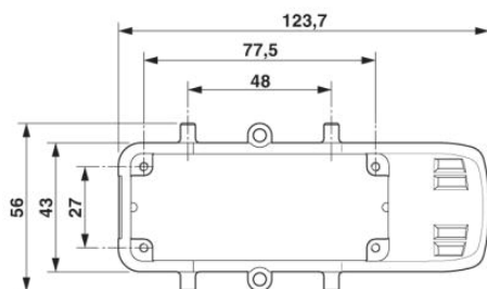
Maatschets bovenaanzicht
