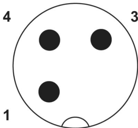
Poolschema stekker M12, 3-polig, A-gepolariseerd, aanzicht stiftzijde
