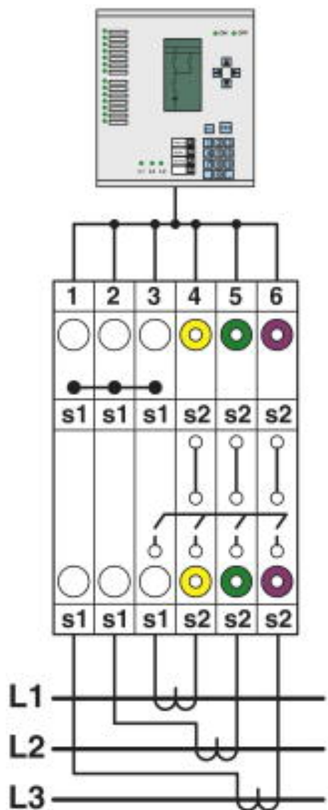
Gekoppelde 3-fase stroomtransformatoren
