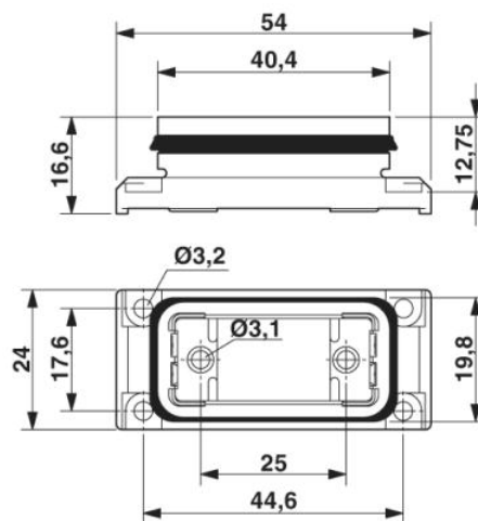
D-SUB-aanbouwraam
