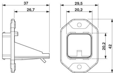
Push-pull-aanbouwraam, Freet- systeem, IP67
