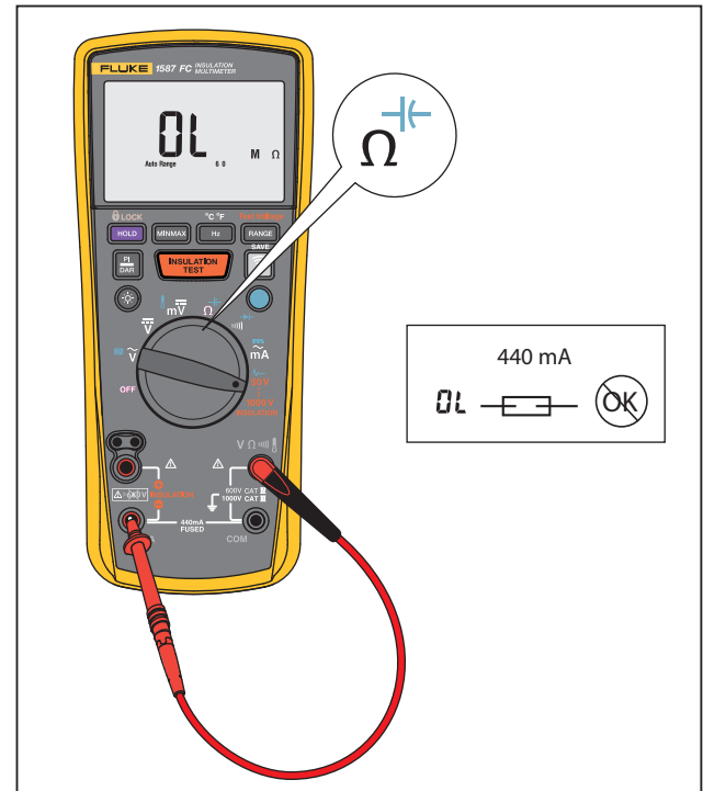
Afbeelding 12. Zekering testen
