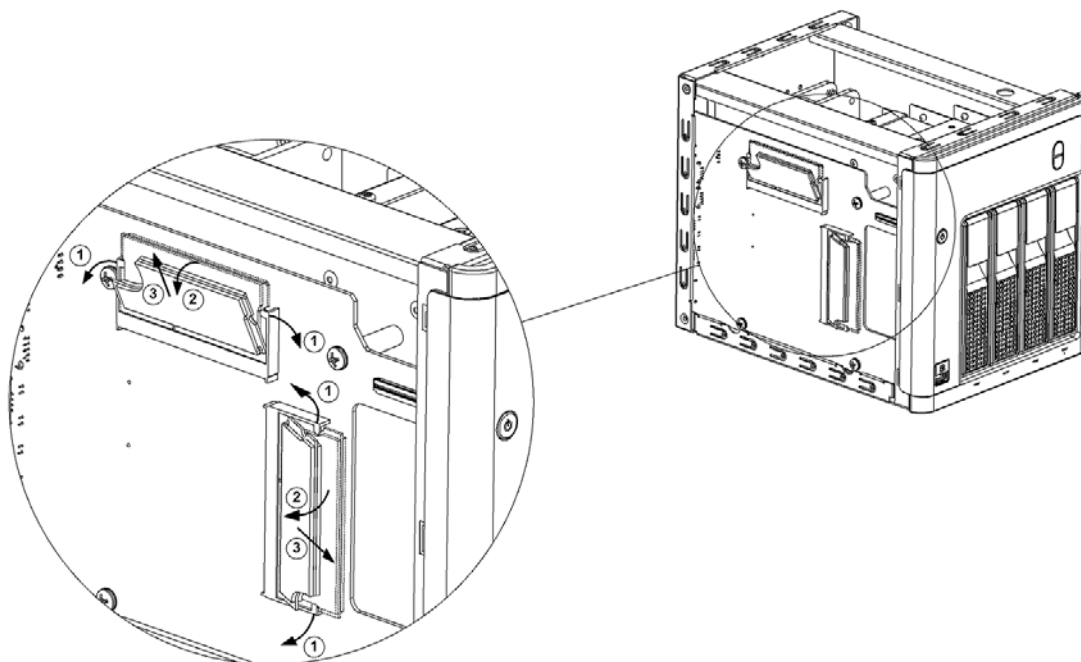
Afbeelding 2. 4PL-SO-DIMM-module vervangen
