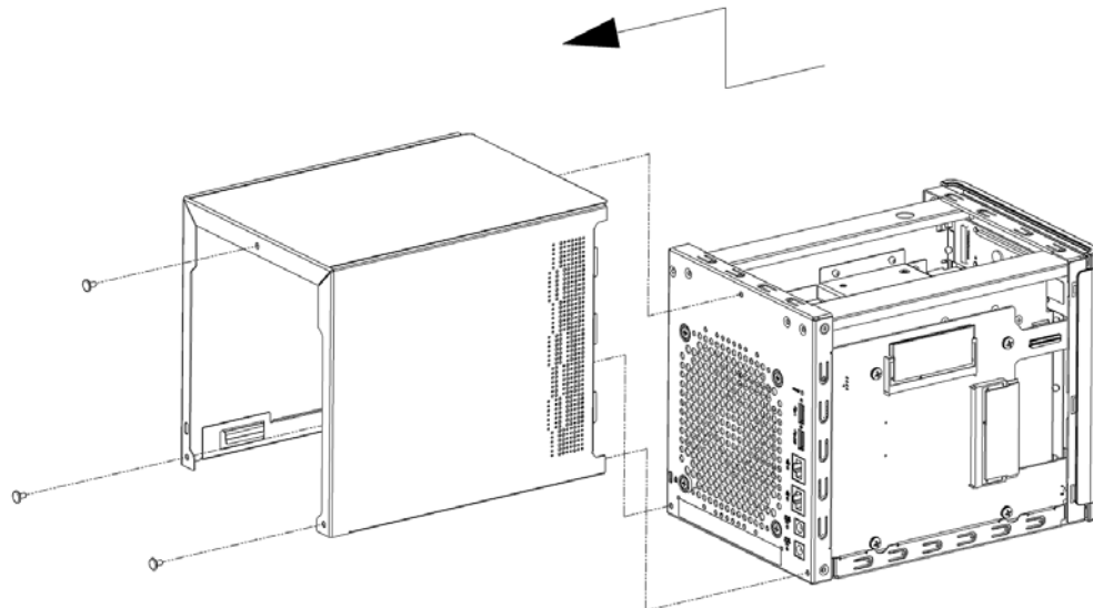
Afbeelding 1. Schroeven losmaken en behuizing verwijderen
