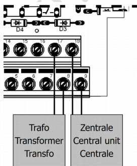
Fig. 3: Stroomtoevoer via een aparte trafo
