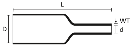
Krimpkous 4:1
