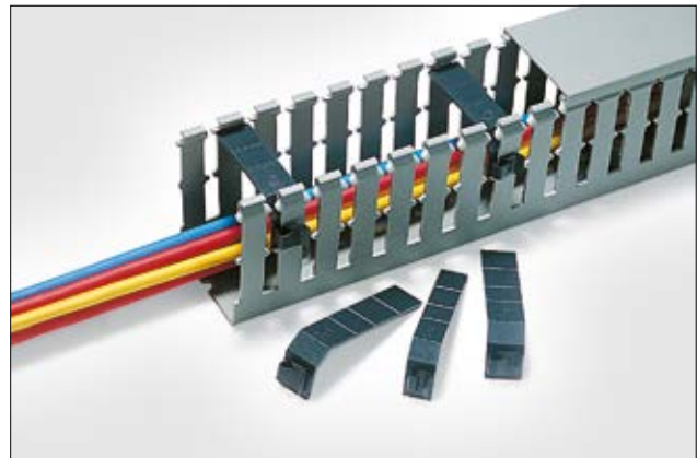
HTWD-NFWR en HTWD-WFWR houden aders op hun plaats als het deksel verwijderd wordt.
