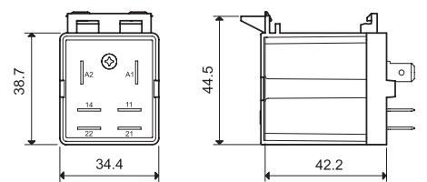
065.08 met relais
