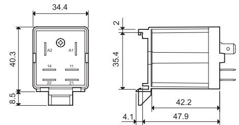
065.07 met relais
